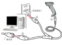
PS2 cables
